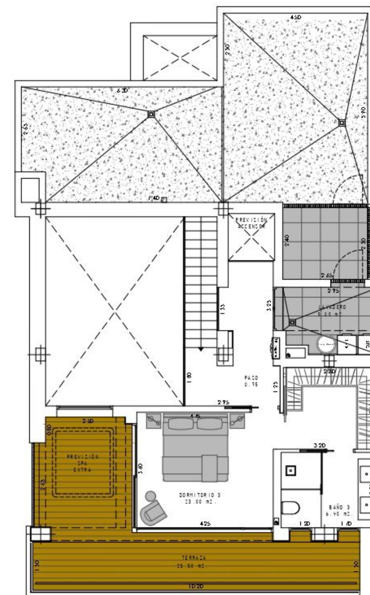
PLANTA ALTA
