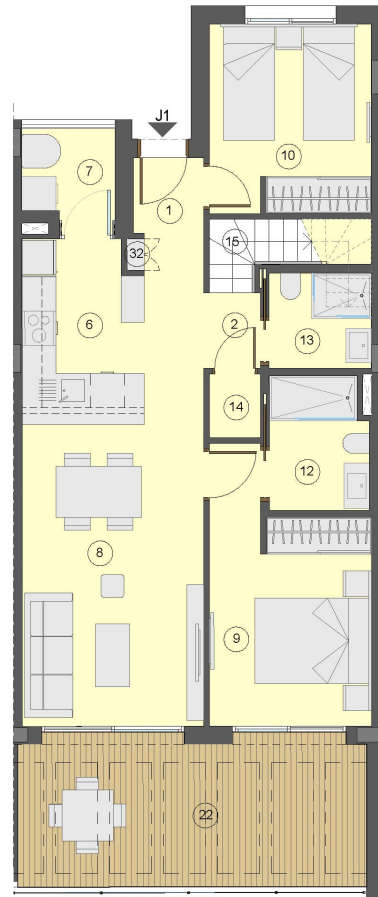
PLANTA PRIMERA
