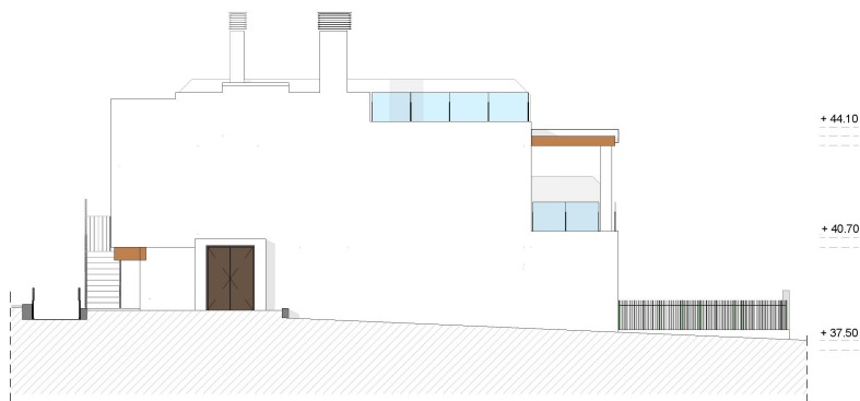
ALZADO SUROESTE
