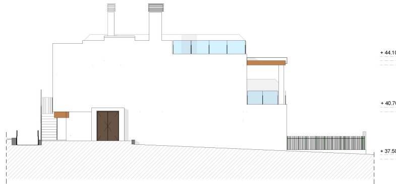
ALZADO SUROESTE
