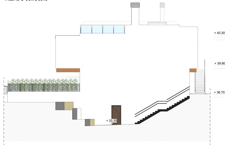
ALZADO NORESTE
