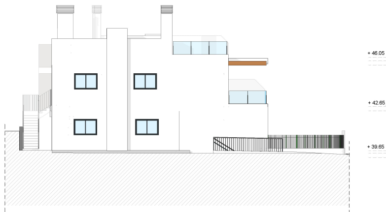
ALZADO SUROESTE
