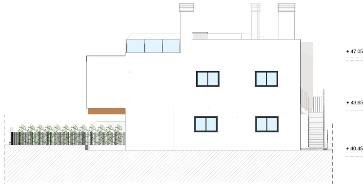
ALZADO NORESTE
