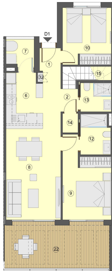
PLANTA PRIMERA
