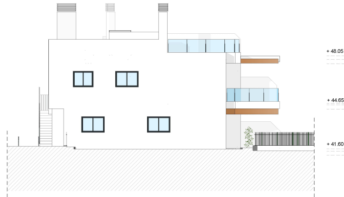
ALZADO SUROESTE
