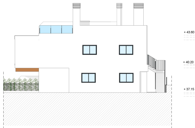
ALZADO SUROESTE
