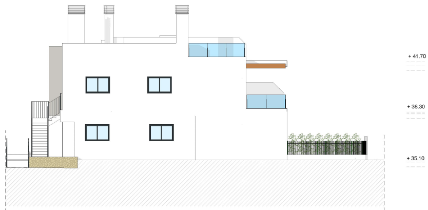
ALZADO NORESTE
