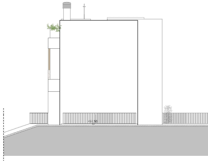
Alzado Norte
