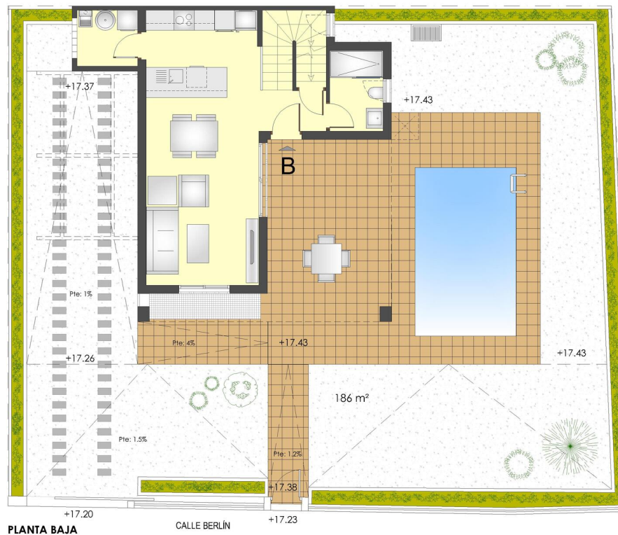
PLANTA BAJA
