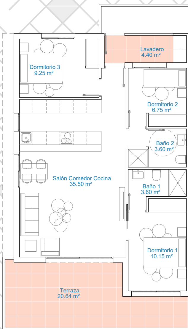
PLANTA PRIMERA
